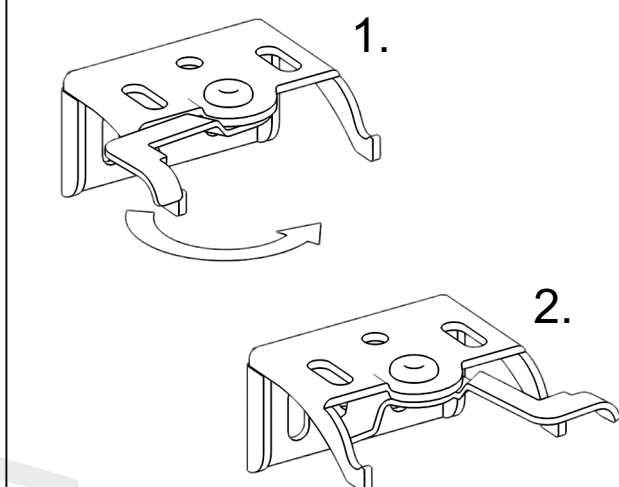
Montaż żaluzji.
