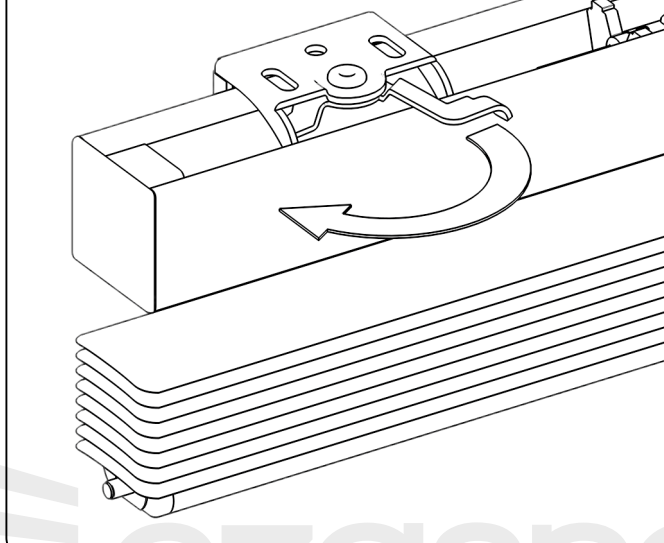
Montaż żaluzji.
