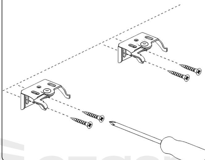
Montaż żaluzji.
