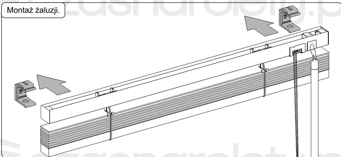
Montaż pokrywy uchwytu.
