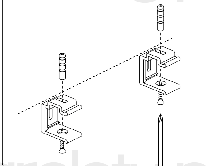
Montaż uchwytych plastikowych - do sufitu.
