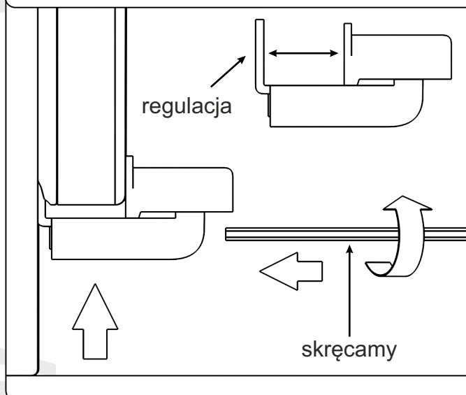
Montaż dolnego bezinwazyjnego uchwyty linki D.
