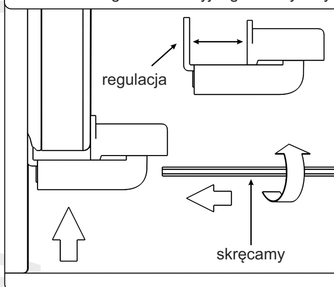
Montaż dolnego bezinwazyjnego uchwyty łyki D.
