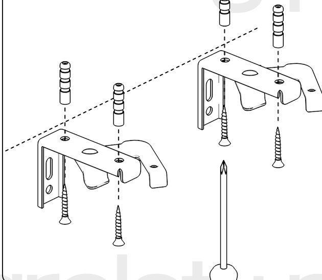
Montaż uchwytych - do sufitu.
